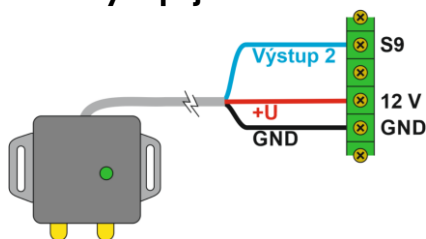
Zapojení s Addat AJK6
